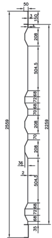
SECTION A-A
